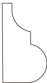
B-69 7/8"x1-9/16"
