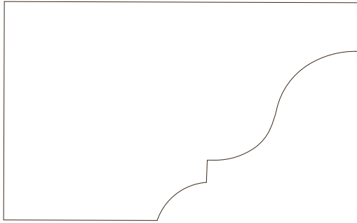
B-73 1-3/8"x2-1/16"
